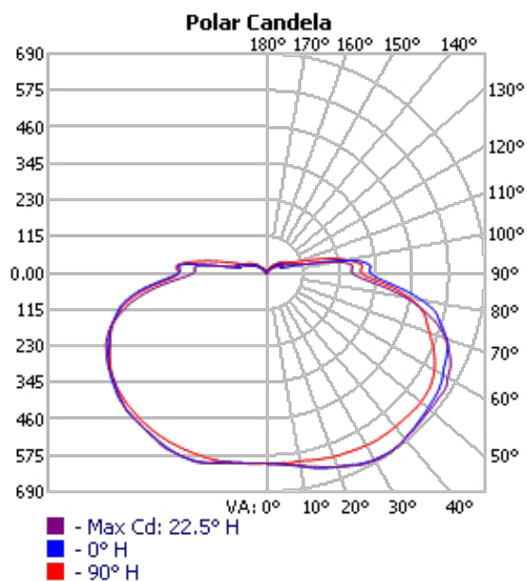
Polar Candela Distribution Distribution polaire de la candela
